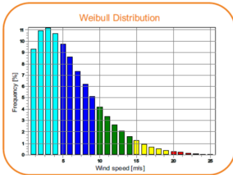
Abbildung 19, Weibull-verteilte Windgeschwindigkeiten
